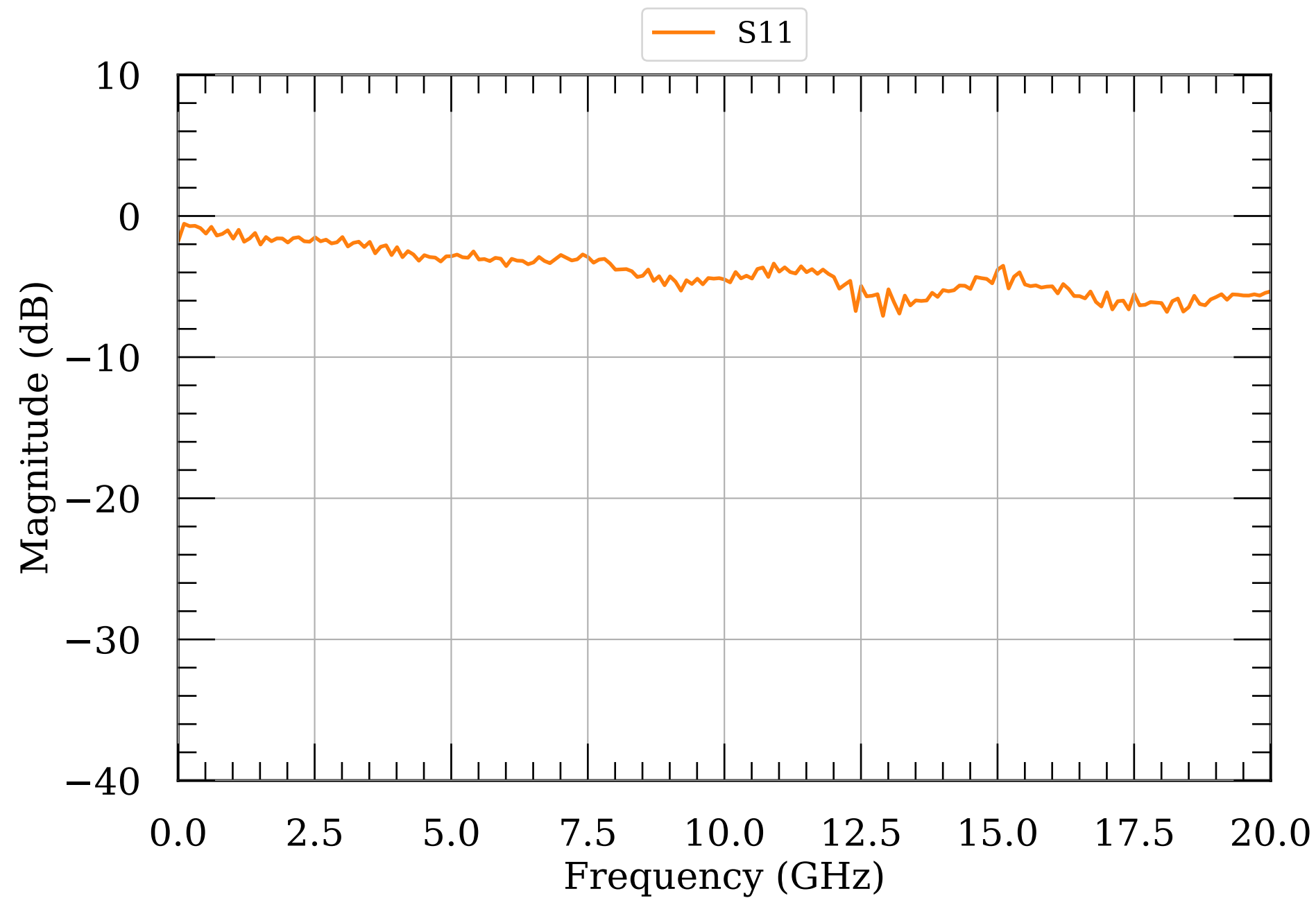
LNA S-params module046
